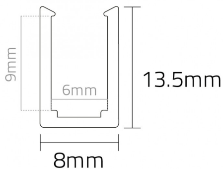
Imagem técnica
